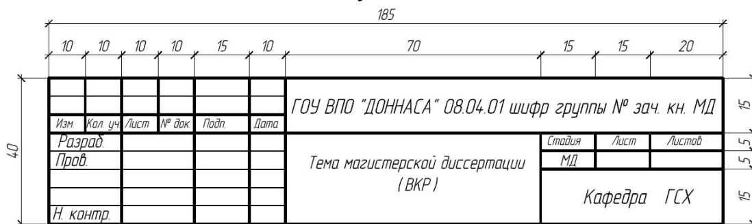
Рисунок 6.2 — Штамп по форме 5 ГОСТ Р 21.1101-2013 для всех видов текстовых документов (первый или заглавный лист)
