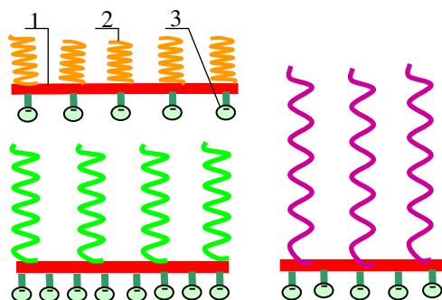
Рисунок 5.6 – Схема строения молекул поликарбоксилатных суперпластификаторов: 1 – основная полимерная цепь; 2 – привитые боковые полимерные цепи; 3 – функциональные
