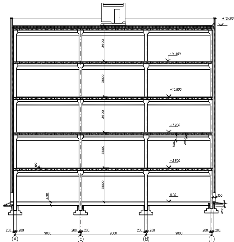
РАЗРЕЗ 1-1
