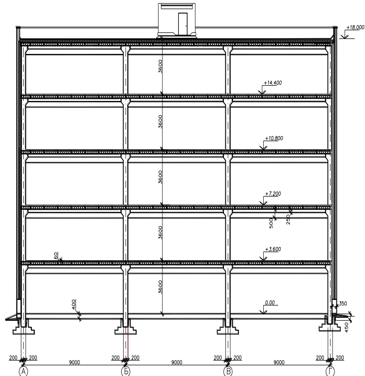
РАЗРЕЗ 1-1
