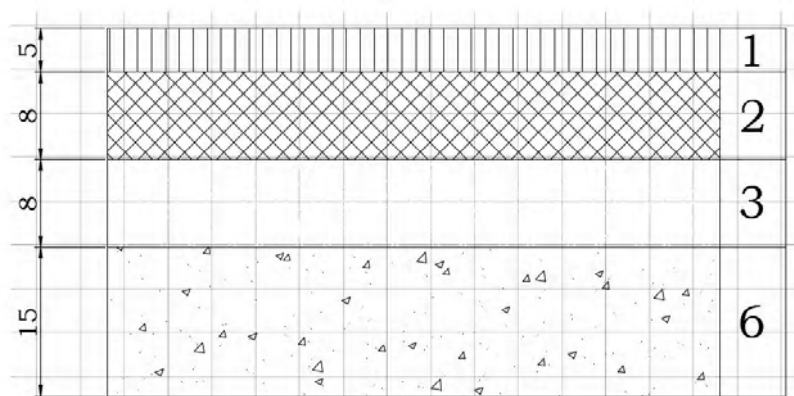
Рисунок 4. Вариант дорожной одежды тип 3.
