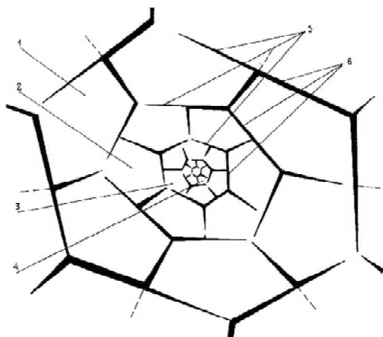
Рис. 2. Модель конструкции в виде общей схемы иерархии активных элементов на различных уровнях структурных неоднородностей: 1 – уровень конструкции (изделия); 2 – уровень бетона; 3 – уровень растворной составляющей (матричный материал на уровне бетона); 4 – уровень цементного камня (матричный материал на уровне раствора); 5 – ТТ; 6 – ВПР.
