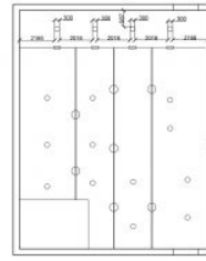
План потолка М 1:100
