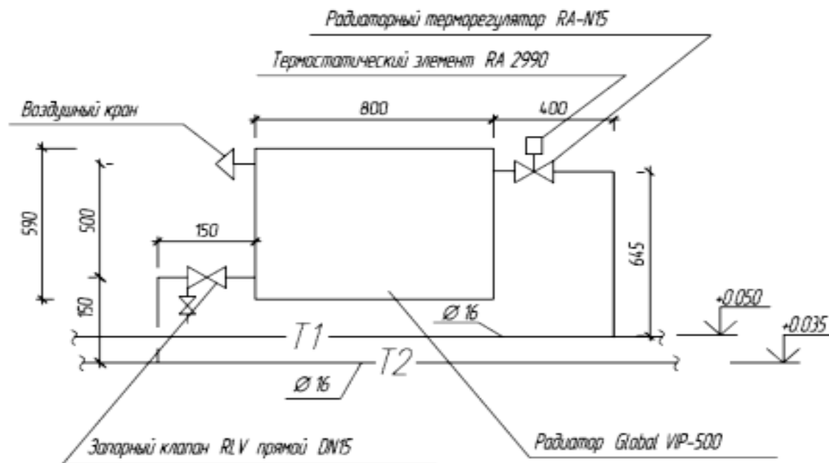
Рисунок 6.1 – Схема подсоединения радиатора
