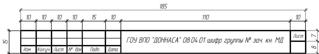
Рисунок 6.3 - Штамп по форме 6 ГОСТ Р 21.1101-2013 для чертежей и всех видов текстовых документов (последующие листы)
