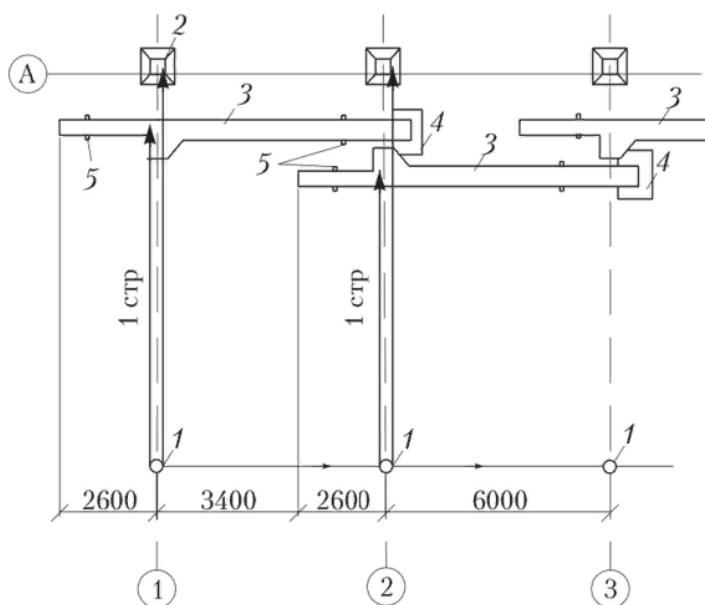
Рисунок 3 - Технологическая схема монтажа колонн способом «скольжения»:
