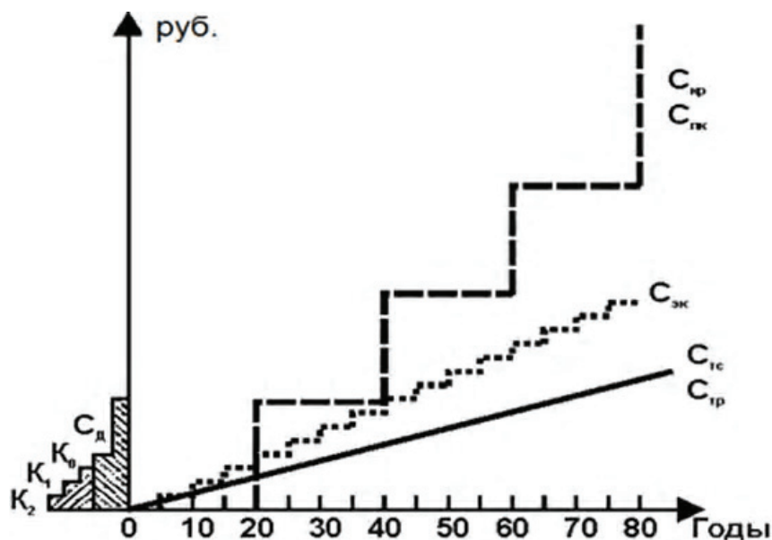
Рисунок – Схематический график учитываемых затрат и издержек: K_0, K_1, K_2 – капитальные вложения в сопряженные отрасли, поставляющие материалы и изделия для строительстве; C_d – затраты при возведении зданий и сооружений; C_{кр} – затраты на капитальный ремонт; C_{эк} – затраты на возобновление защиты от коррозии; C_{тр} и C_{мс} – среднегодовые затраты на текущий ремонт и содержание; C_{ПК} – потери от коррозии при эксплуатации зданий и сооружений.
